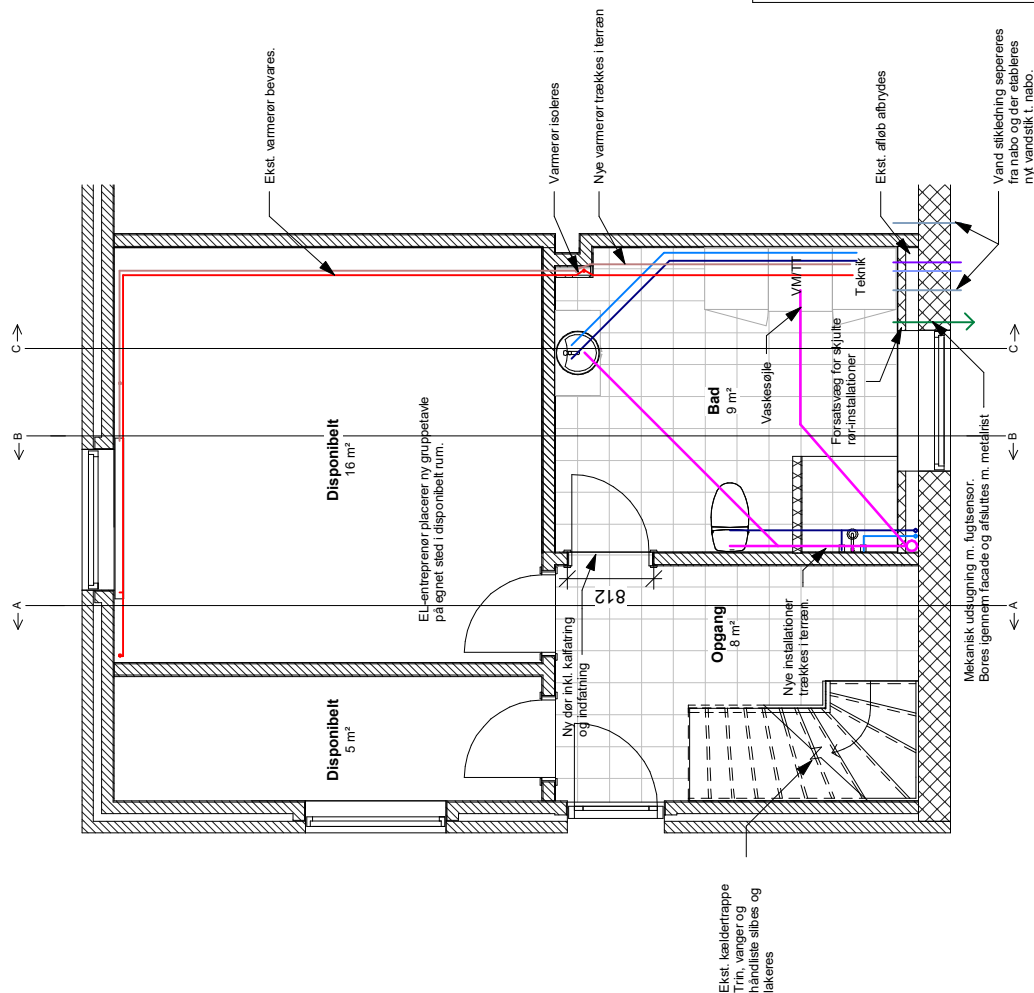
-01 - Kælderplan | 1 : 50
